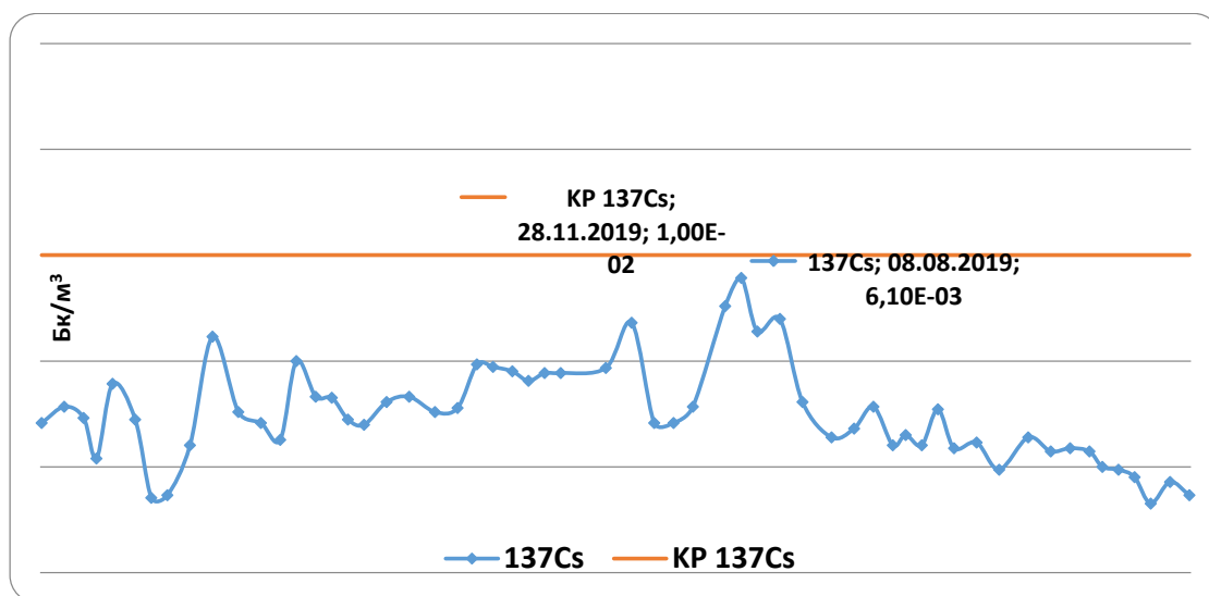
Динаміка об'ємної активності (Бк/м 3 ) ^{137}\text{Cs} в приземному шарі повітря на АСКРС ВРП-750 у 2019 році
