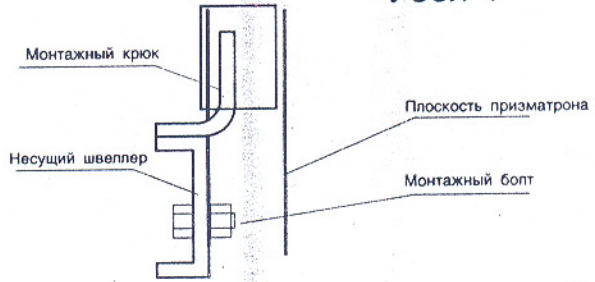
Узел I
