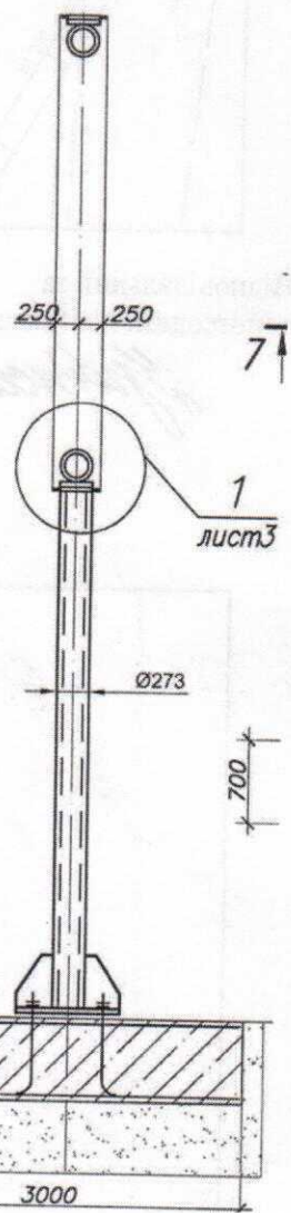
1-1 M1:50
