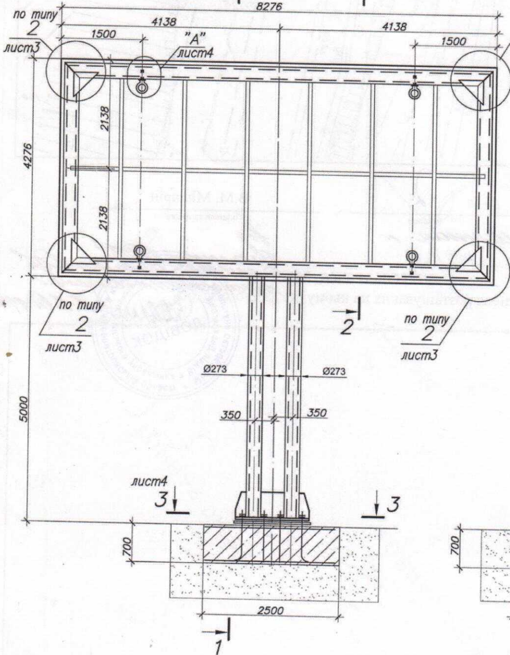
Общий вид лист 4 1 M1:50 2
