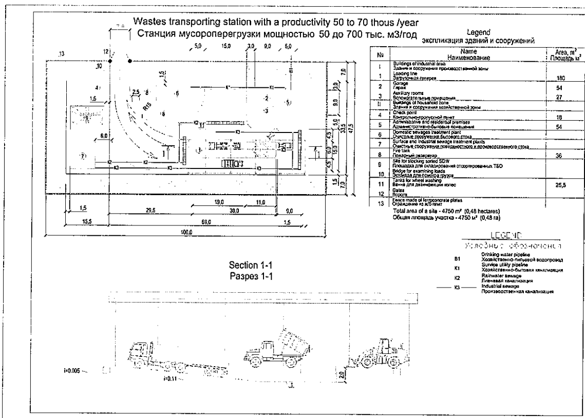
Рис. 1. Станція перевантаження сміття потужністю 50 – 70 тис. куб. м/рік
