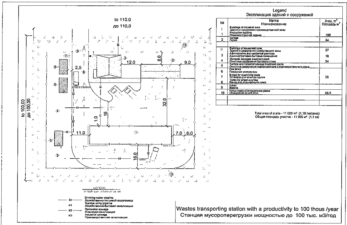
Рис. 3. Станція перевантаження сміття потужністю 100 тис. куб. м/рік
