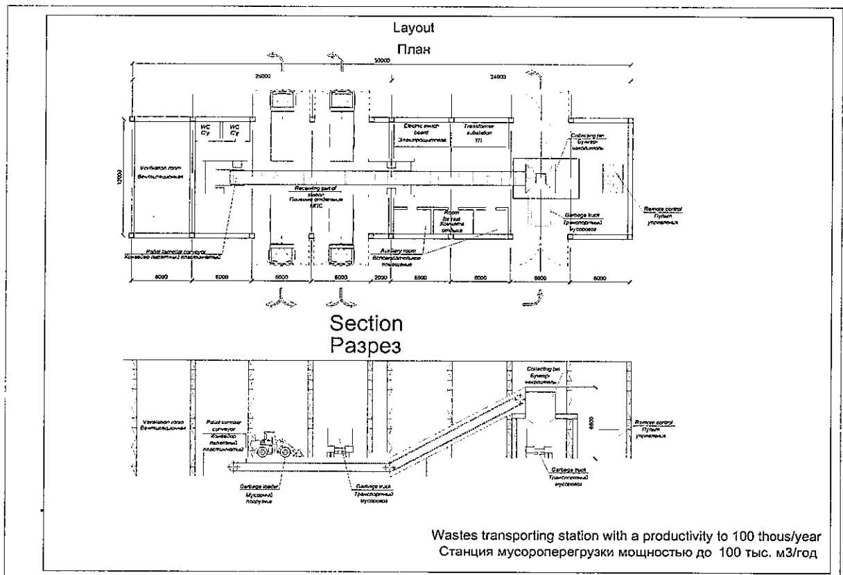
Рис. 3. Станція перевантаження сміття потужністю 100 тис. куб. м/рік
