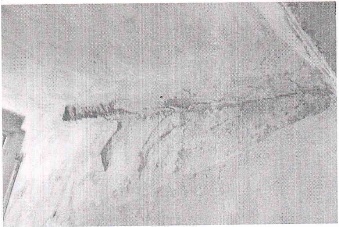
Фото В.8. Приміщення №80, відшарування захисного шару бетону косоура сходового маршу с голенням кородуючої робочої арматури
