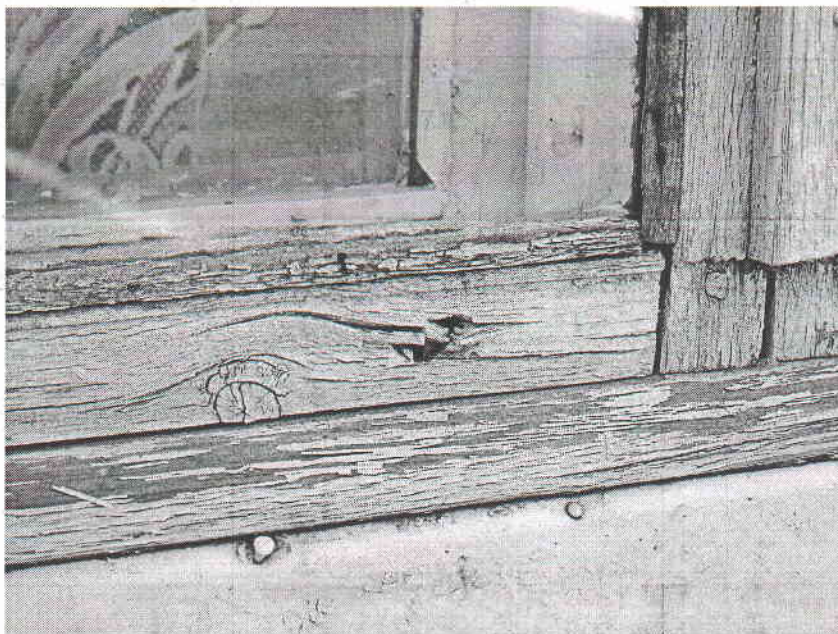
Рис.2. Повреждение части древесины оконных рам гнилью, грибком, насекомыми вплоть до полного отсутствия каркаса
