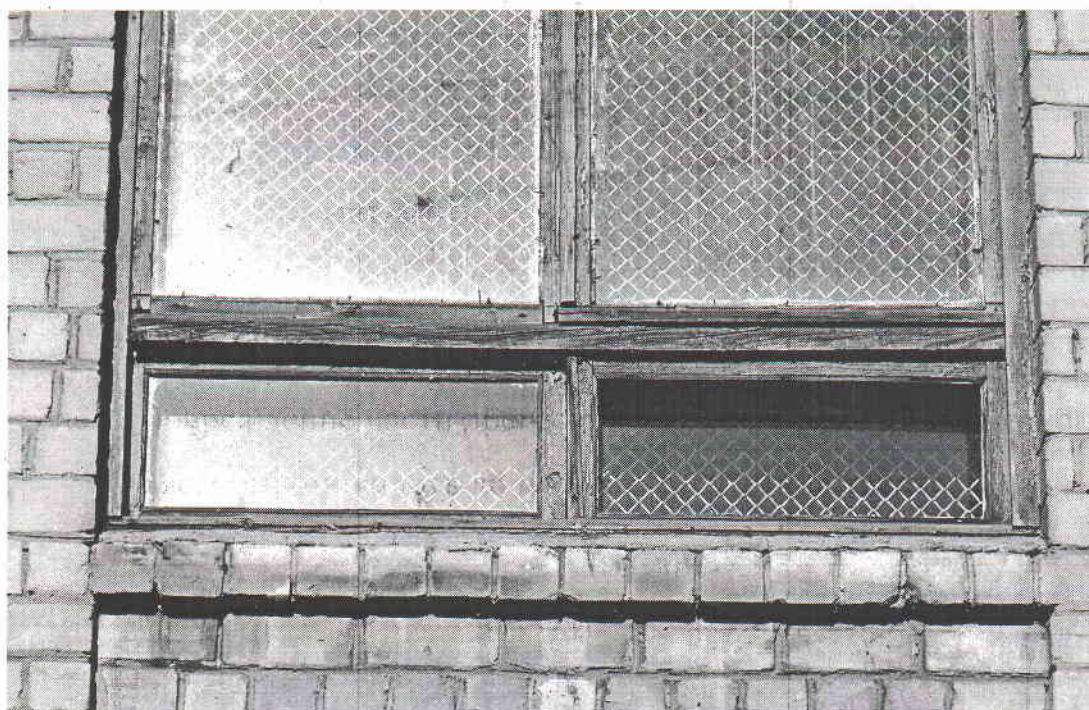
Рис. 3. Повреждение и отсутствие штапиков крепления наружных стекол
