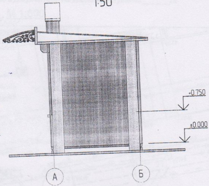
Фасад А-Б
