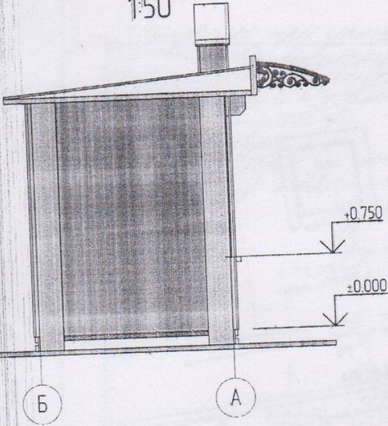
Фасад Б-А
