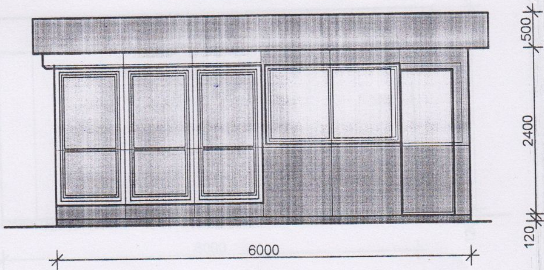
Головний фасад ТС М 1:50
