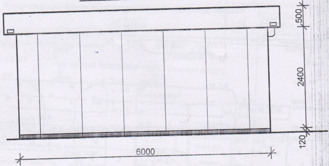
Боковий фасад ТС М 1:50
