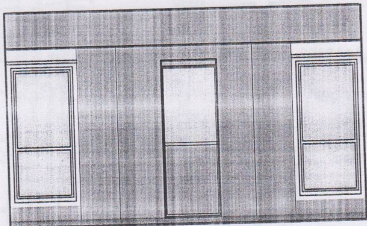
Боковий фасад ТС М 1:50
