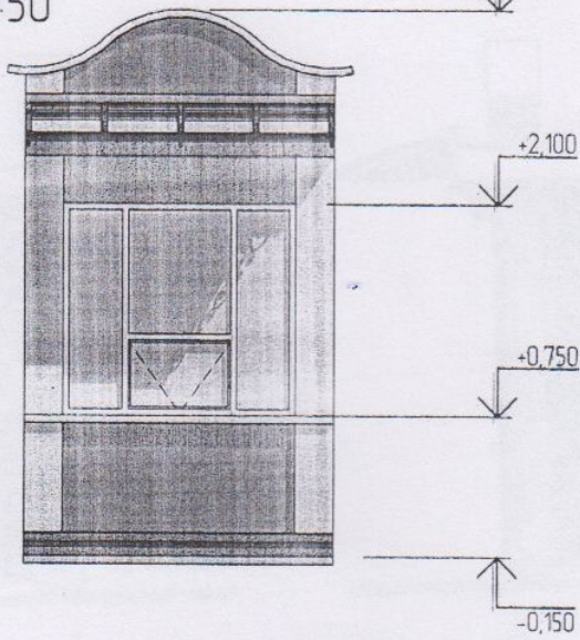
Фасад 1-2
