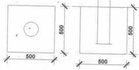
Фундамент під ворота
