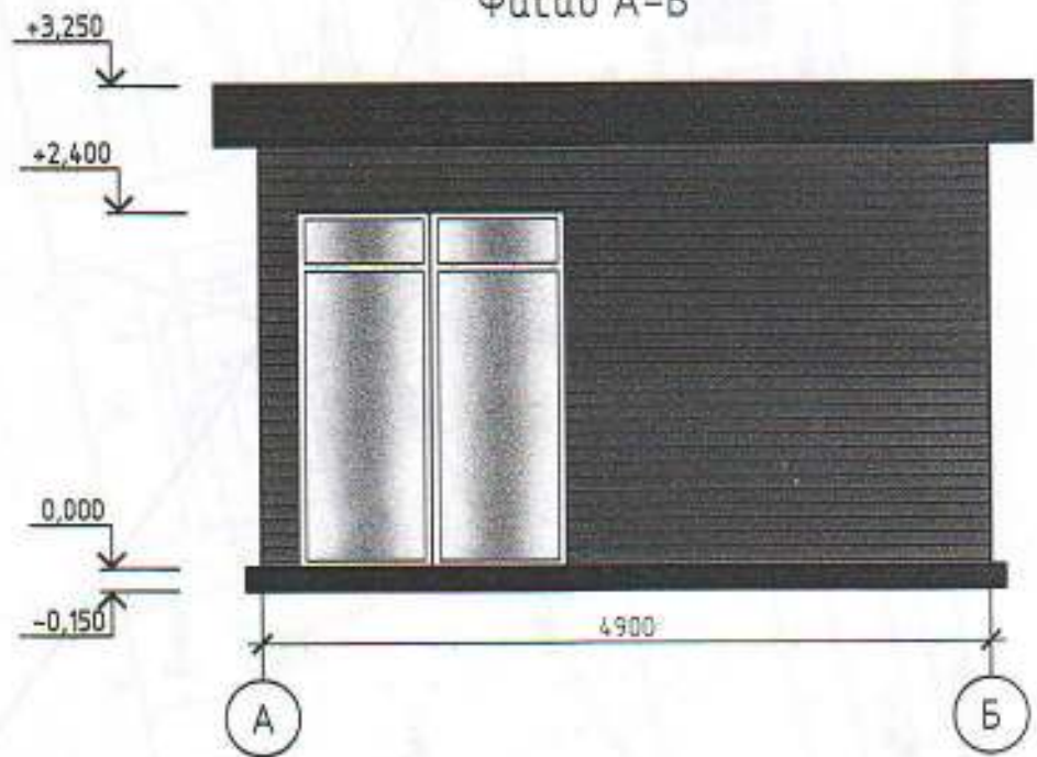
Фасад А-Б
