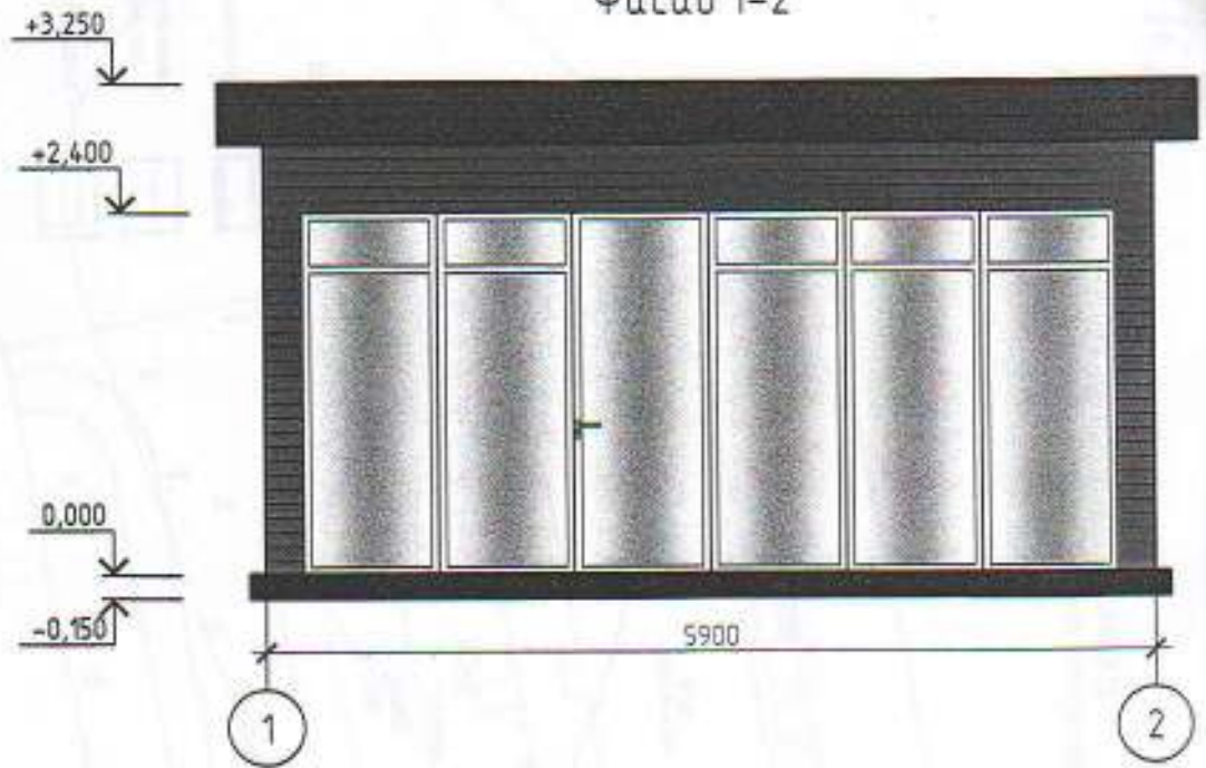
Фасад 1-2
