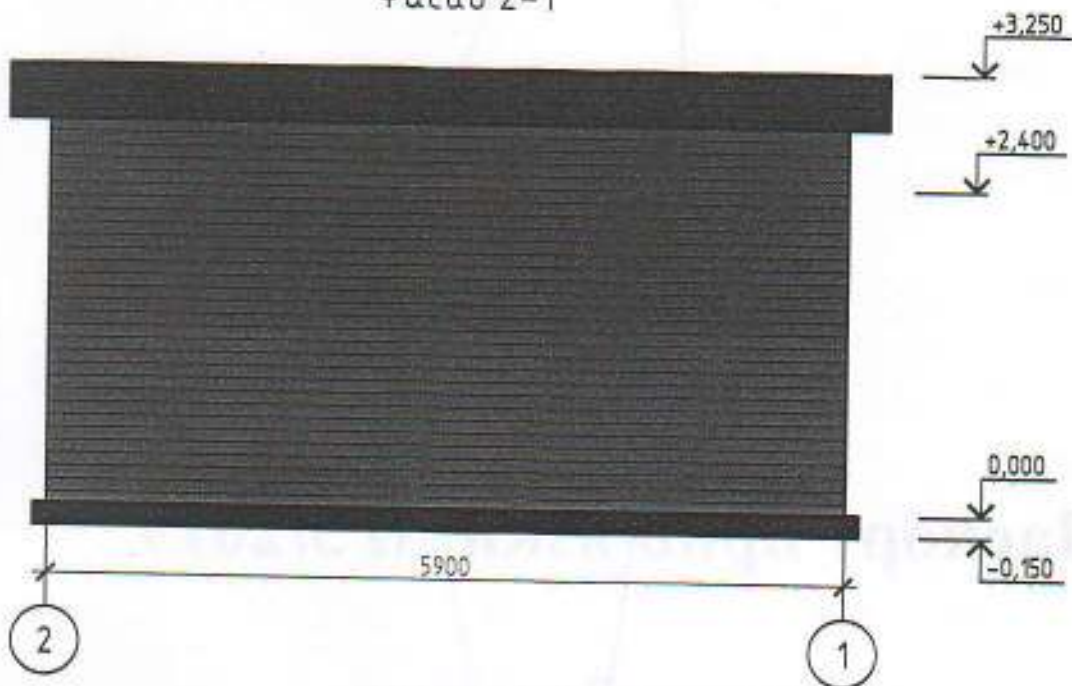
Фасад 2-1
