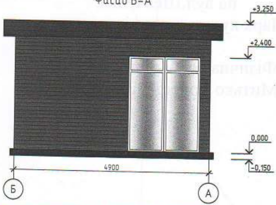
Фасад Б-А
