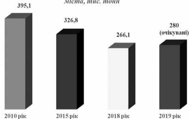
Обсяги викидів забруднюючих речовин в атмосферне повітря міста, тис. тонн
